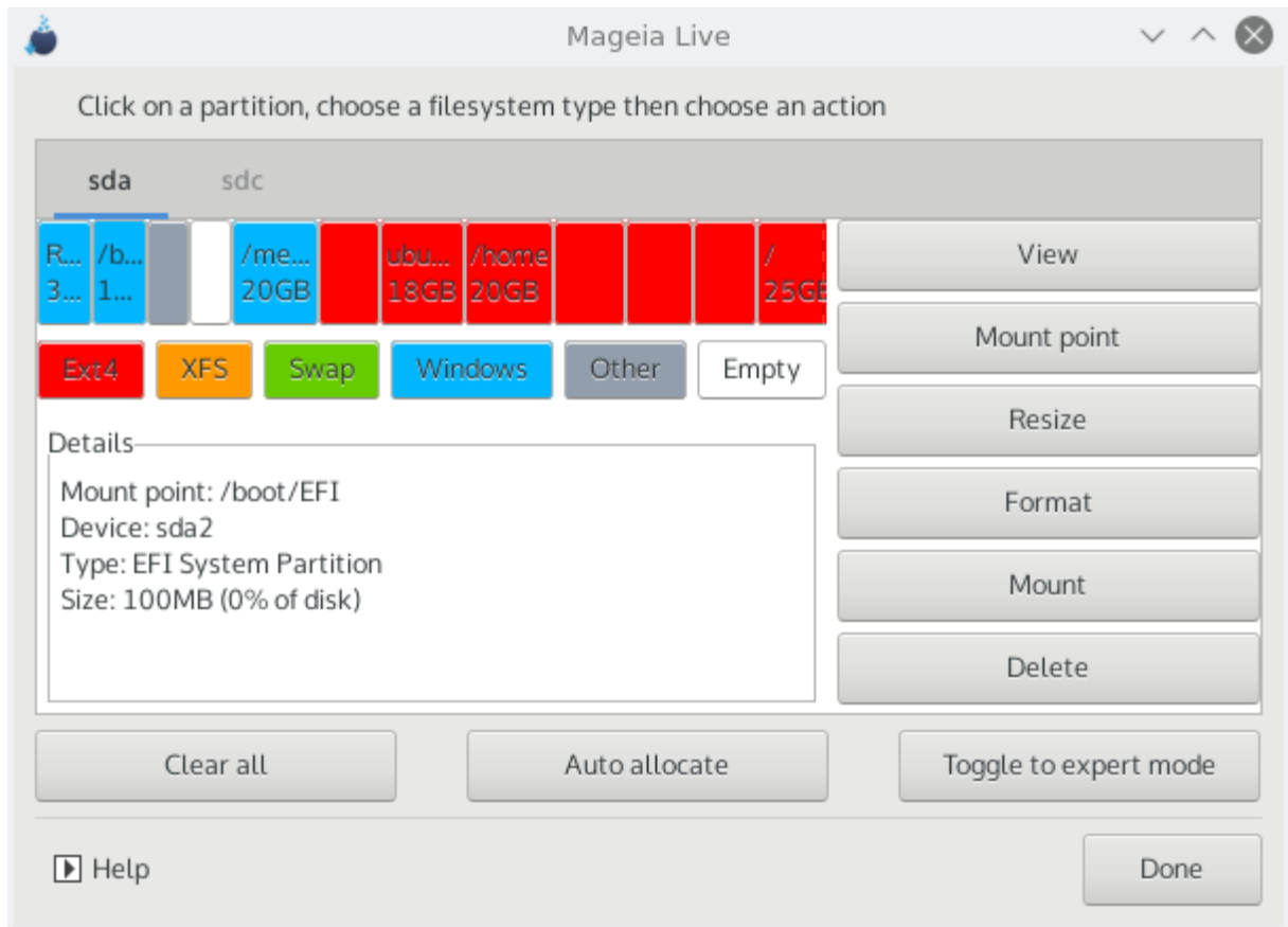
Abbildung 1. EFI-Systempartition
